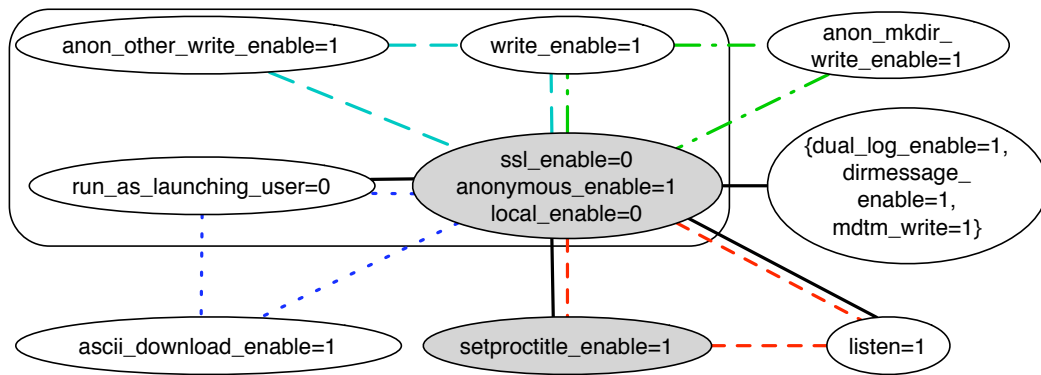
(b) vsftpd
